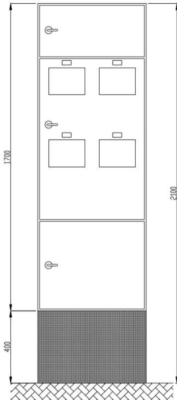
Em pedestal de alvenaria
